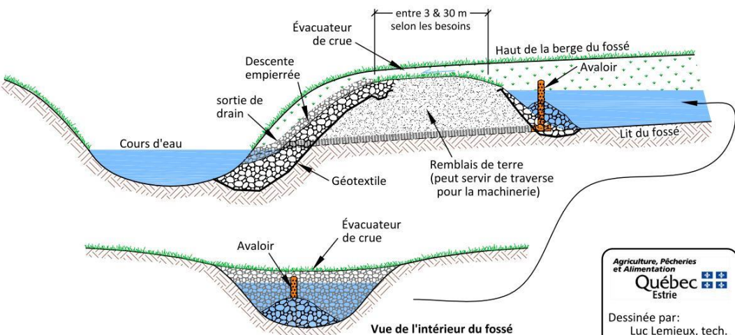
Figure 2 Construction d'un seuil
